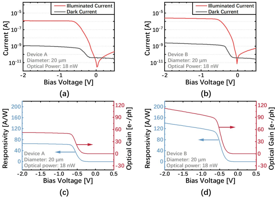
图3 (a)器件A和(b)器件B在室温下有无1.55μm光照的IV曲线以及(c)器件A和(d)器件B的响应度和光学增益曲线
