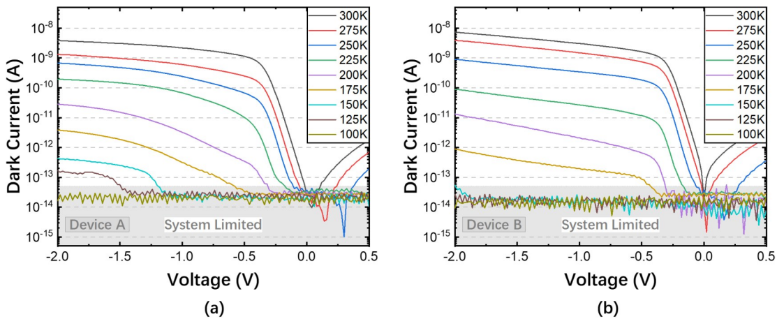
图4 100~300 K温度下(a)器件A与(b)器件B的暗电流-电压曲线
