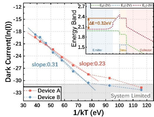
图5 器件A和器件B在-2 V偏压下不同温度暗电流曲线对比
