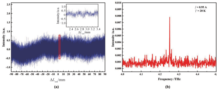
图6 基于自混合效应的闪耀光栅表征结果: I=0.95 A时,(a)加入光栅后THz QCL的自混合干涉时域信号;(b)频谱图
