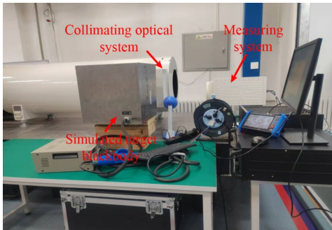
Fig. 1 Experimental setup 图1 试验布置
