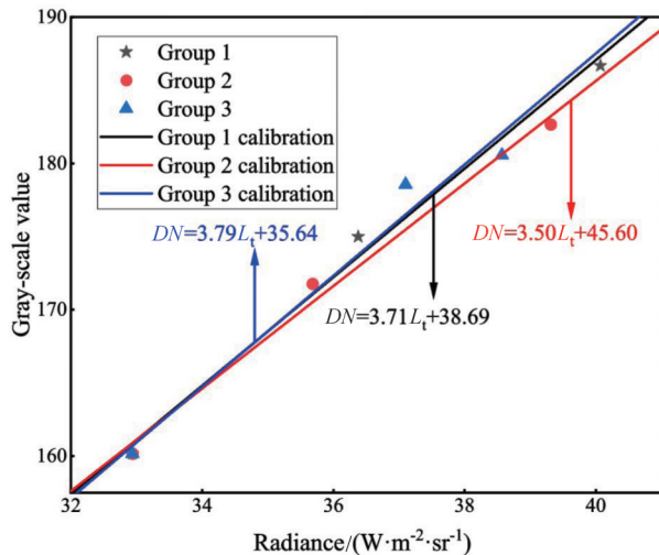
Fig. 4 Calibration curve 图4 标定曲线
