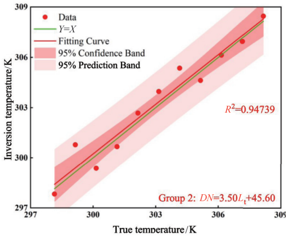
Fig. 6 Group 2 regression analysis 图6 标定组2回归分析
