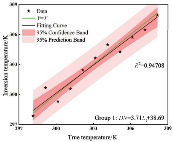
Fig. 5 Group 1 regression analysis 图5 标定组1回归分析
