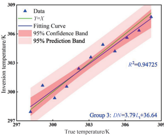
Fig. 7 Group 3 regression analysis 图7 标定组3回归分析
