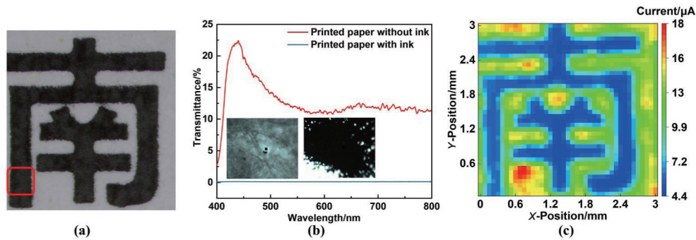
图5 打印的“南”字,有墨区与无墨区的透射光谱与光电流图像:(a)小五号字体打印的“南”字;(b)有墨区和无墨区的透射光谱,插图为对应的显微照片;(c)控制器1600细分扫描的光电流图像
