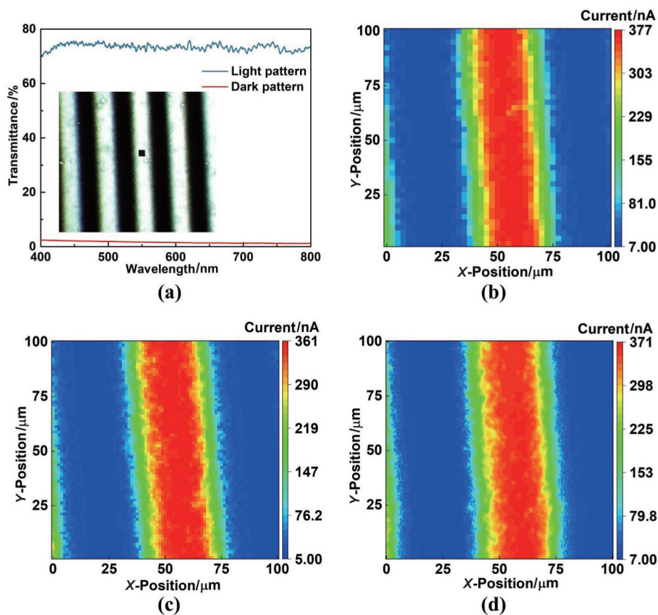
图7 光栅条亮区和暗区的透射光谱曲线及不同扫描步长下覆盖光栅条的硅太阳能电池的光电流扫描结果:(a)光栅条亮区和暗区的透射光谱曲线,插图为其显微照片;(b)2.5 \mu\text{m} 步长;(c)1.25 \mu\text{m} 步长;(d)0.625 \mu\text{m} 步长
