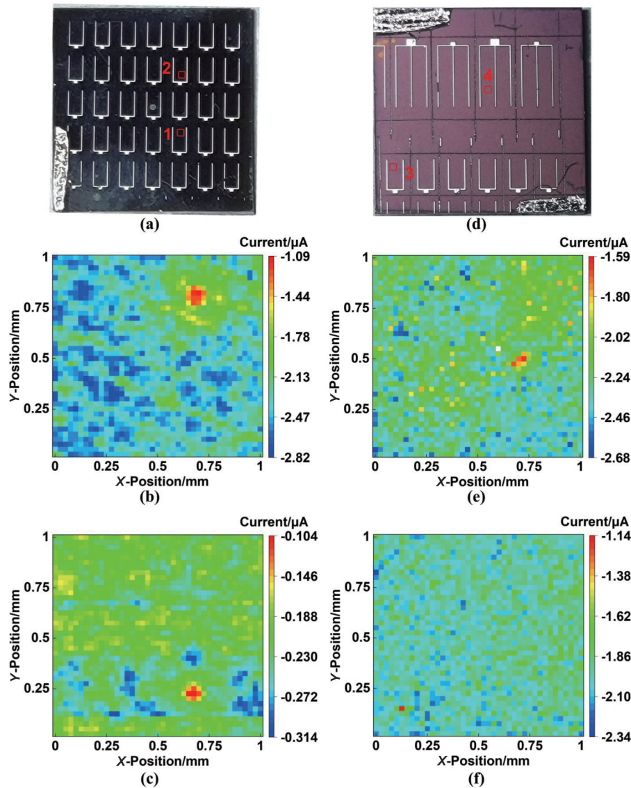
图8 \text{Cu}_2\text{ZnSnS}_4 和 \text{Cu}_2\text{ZnSn}(\text{S}, \text{Se})_4 太阳能电池实物图及光电流扫描图像:(a) \text{Cu}_2\text{ZnSnS}_4 太阳能电池样品实物照片;(b)电池1的光电流图像;(c)电池2的光电流图像;(d) \text{Cu}_2\text{ZnSn}(\text{S}, \text{Se})_4 太阳能电池样品实物照片;(e)电池3的光电流图像;(f)电池4的光电流图像
