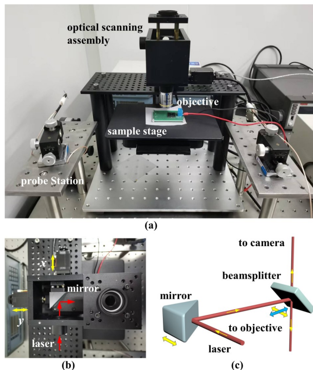
图1 研制的光电流 mapping 系统:(a)实物图;(b)由光学组件组成的光束扫描组件的内部结构;(c)光束扫描组件的内部光路示意图
