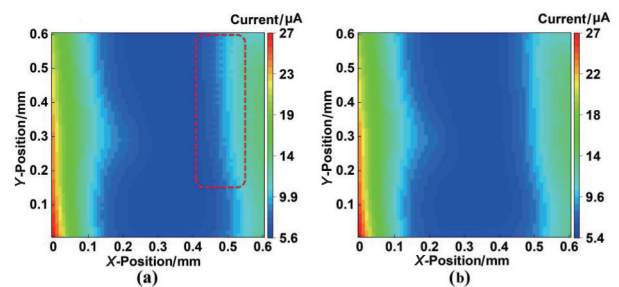
图6 打印的“南”字左下角竖直部分的光电流图像:(a)S型扫描;(b)单向扫描
