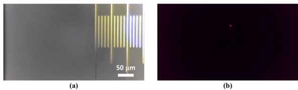
图2 相机拍摄的聚焦图像与光斑:(a)10 μm 间隔的测微尺;(b)聚焦光斑
