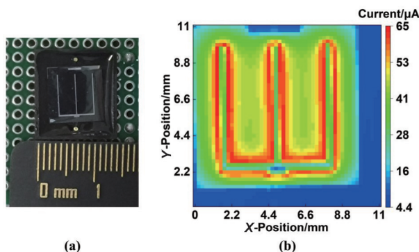
图4 硅光电池实物图和光电流图像:(a)硅光电池;(b)硅光电池的光电流图像
