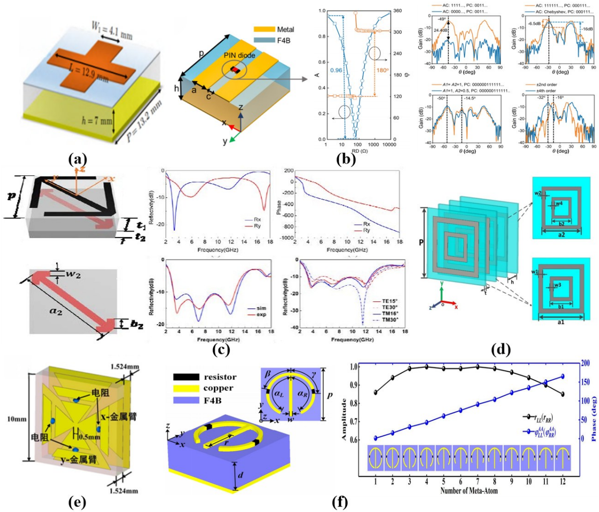
图7 (a)单层柔性超表面单元 [90] ;(b)超表面单元,10 GHz下从 1 \Omega 到 10000 \Omega 时单元的反射幅值和相位仿真结果,四种不同的幅值-相位联合编码序列测量的超表面的二维远场辐射模式 [91] ;(c)双层箭头超表面单元结构,单元相位和幅值仿真结果,实测与仿真结果对比结果 [92] ;(d)超表面单元 [93] ;(e)超表面单元 [93] ;(f)超表面单元及其在10.0 GHz频率的工作幅值相位的仿真结果 [94]
