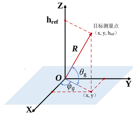
图4 激光雷达极坐标和测量点坐标投影
