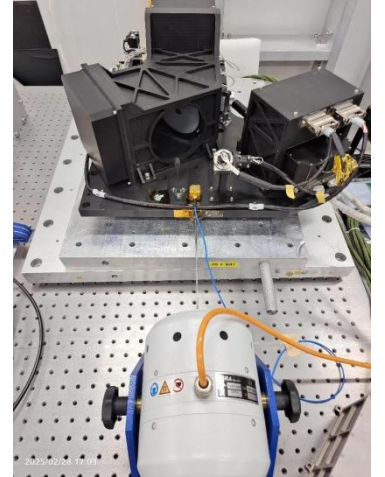
Fig. 5 The experimental platform 图5 实验平台
