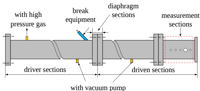
图5 激波管结构示意图 Fig. 5 Schematic diagram of shock tube structure
