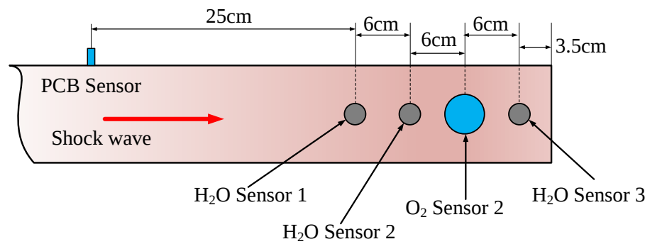
图8 光学探头安装相对位置示意图 Fig. 8 Schematic Diagram of the Relative Position of Optical Probe Installation
