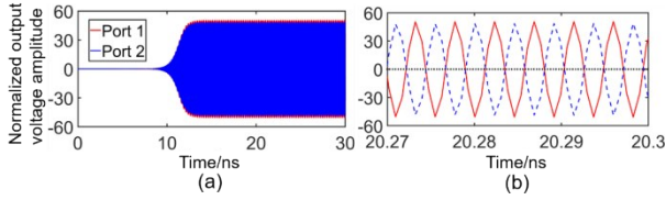
图 13 当耦合桥长为 L_g 的振荡器被电压 23 kV 下一个电流为 0.6 A 且另一个电流为 0.4 A 的双电子注驱动时,该图表示(a)两个端口的输出信号;(b)用于显示相位差的 20.27 ns 到 20.3 ns 之间信号的详细信息
