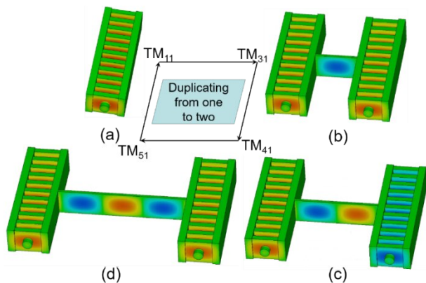
图2 典型模式纵向电场( E_z 场)的三维分布图,模式包括(a)传统单个扩展相互作用电路中 TM_{11} 模;具有不同 L_g 共谐振电路系统的(b) TM_{31} 模;(c) TM_{41} 模;(d) TM_{51} 模
