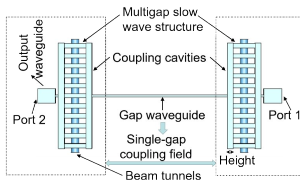
图1 基于共谐振电路系统的双电子注振荡器模型示意图
