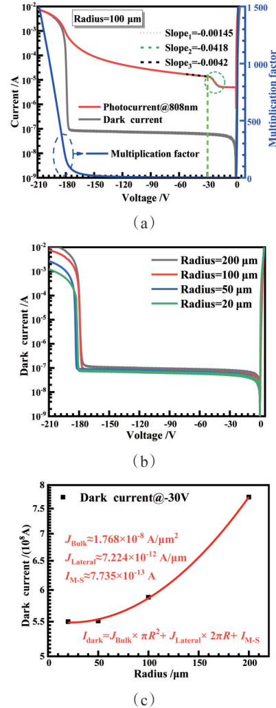
图3 SACM型APD的 I - V 特性及不同尺寸暗电流特性:(a)尺寸为100 \mu\text{m} 的SACM型APD的 I - V 特性和倍增系数;(b)光敏面半径为20 \mu\text{m} 、50 \mu\text{m} 、100 \mu\text{m} 、200 \mu\text{m} 器件的暗电流曲线;(c)-30 V偏压下暗电流与光敏面半径的关系,红线是根据公式(1)的拟合曲线
