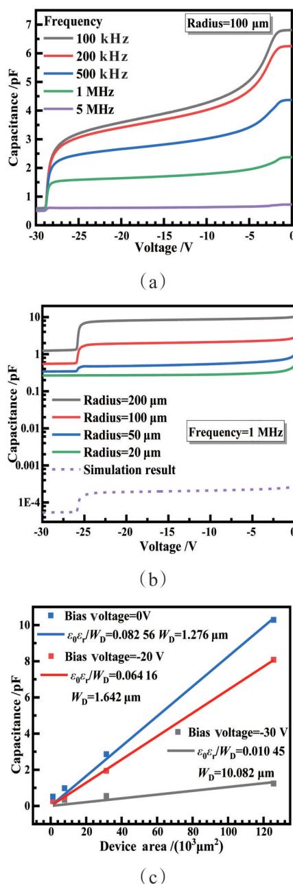
图5 SACM型APD的C-V特性:(a)在100 kHz、200 kHz、500 kHz、1 MHz、5 MHz频率下100 \mu\text{m} SACM型APD的C-V特性;(b)1 MHz下不同光敏面半径器件的C-V特性(虚线为半径100 \mu\text{m} 器件在1 MHz频率下电容仿真曲线);(c)器件在0 V、-20 V、-30 V偏压下的电容值与器件光敏面面积拟合关系
