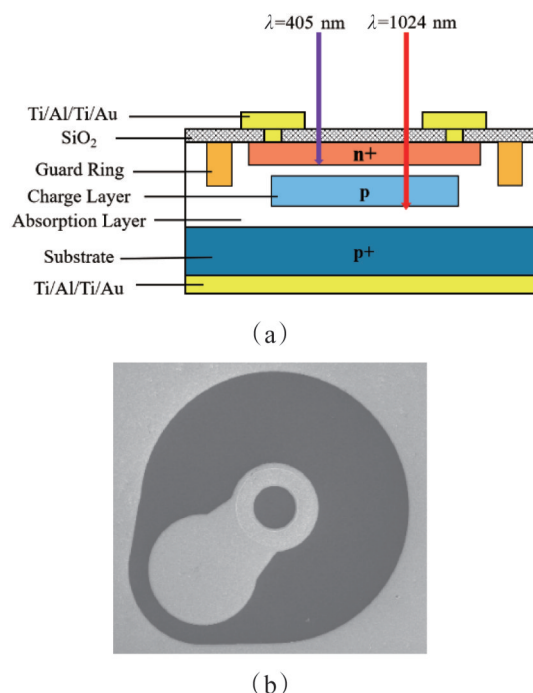
图 1 器件结构示意图:(a) SACM 型 APD 结构剖视图;(b) SEM 图
