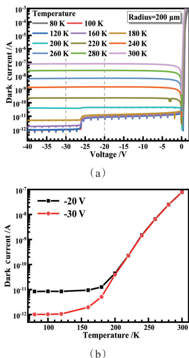
图6 SACM型APD的温度特性:(a)不同温度下尺寸为200 μm的SACM型APD的暗电流特性;(b)-20 V和-30 V偏压下器件暗电流随温度的变化关系
