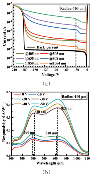
图 4 SACM 型 APD 的 I - V 光电流特性及光谱响应:(a) 尺寸为 100 μm 的 SACM 型 APD 在不同波长下的 I - V 特性;(b) 尺寸为 100 μm 的 SACM 型 APD 在不同偏压下的光谱响应
