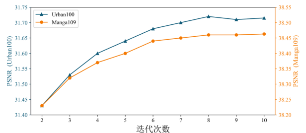
图5 在Urban100和Manga109数据集上PSNR值随迭代数变化曲线 Fig. 5 PSNR values variation curve with iterations on Urban100 and Manga109 datasets
