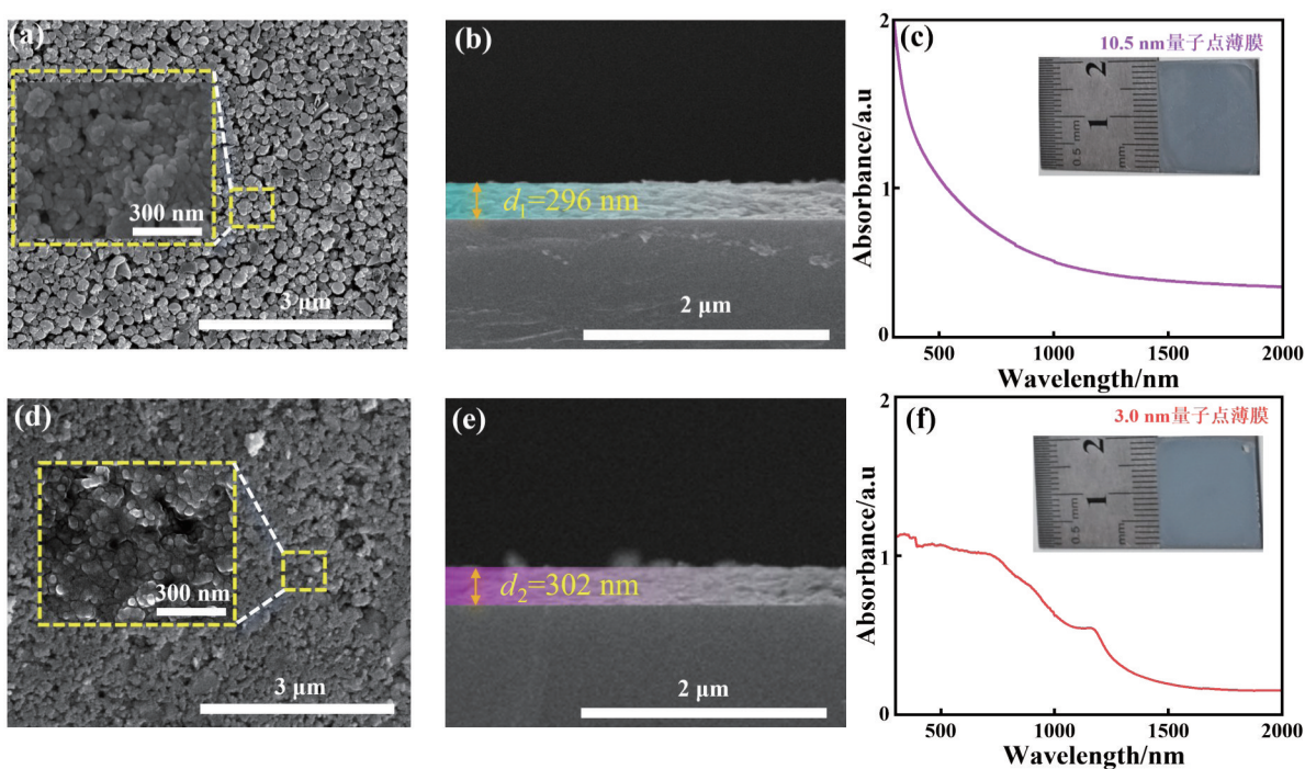
图3 MoTe 2 量子点薄膜的SEM和UV-Vis-NIR吸收光谱:量子点薄膜俯视SEM图:(a)粒径10.5 nm,(d)粒径3.0 nm;量子点薄膜断面SEM图:(b)粒径10.5 nm,(e)粒径3.0 nm;量子点薄膜UV-Vis-NIR吸收光谱:(c)粒径10.5 nm,(f)粒径3.0 nm,插图为薄膜照片
