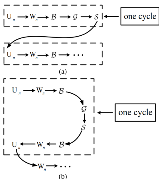
图2 ADMM算法和sGSADMM算法的比较:(a) ADMM算法;(b) sGSADMM算法
