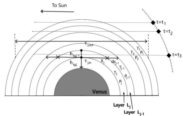
图1 太阳掩星观测示意图
