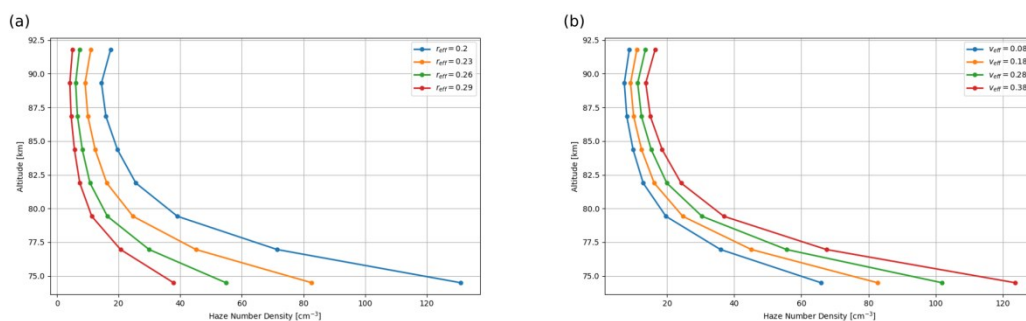
图 18 2006 年 9 月 9 日 (order 149 orbit 141) 金星上层霾数密度随有效半径 r_{eff} 和有效方差 v_{eff} 的变化: (a) 数密度随有效半径 r_{eff} 的变化; (b) 数密度随有效方差 v_{eff} 的变化
