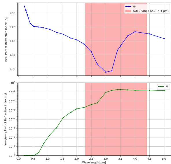
图8 75% H_2SO_4 的折射率在温度 T = 220 \text{ K} 时的复折射率。SPICAV SOIR 光谱范围用阴影表示
