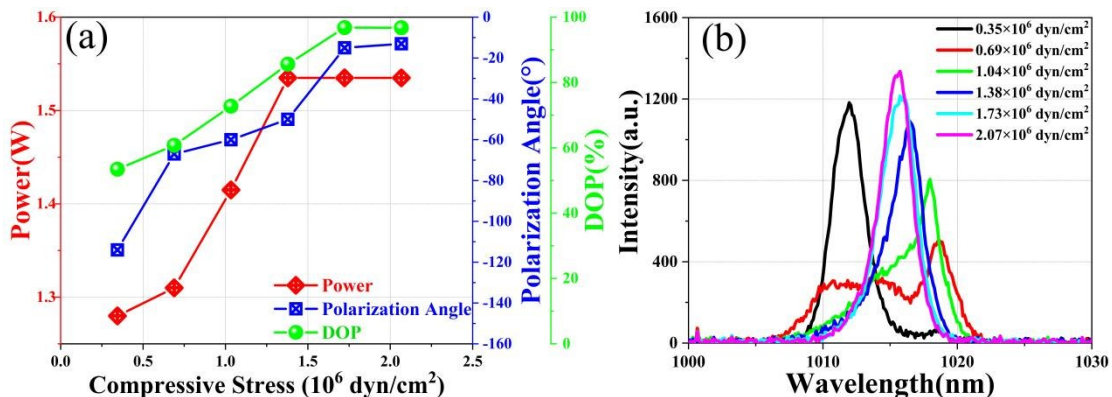
图3 (a)锥形波导的功率、偏振角度与水平夹角、偏振度随压力的变化曲线;(b)锥形波导激光光谱随压力变化情况
