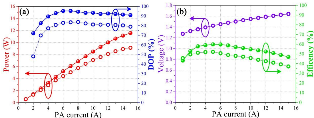
图 5 改善前、后 MOPA 器件的(a)功率、偏振度和(b)电压、转换效率随偏置电流的变化曲线
