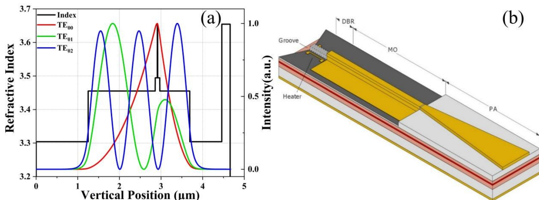
图 1 (a) 980 nm 半导体激光器的折射率、光场分布图;(b) MOPA 器件结构示意图
