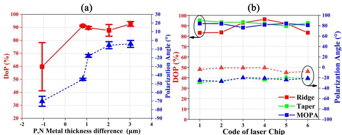
图4 (a)PN金属厚度差对MOPA偏振度、偏振角度的影响;(b)脊型、锥形、MOPA器件的偏振度与偏振角度
