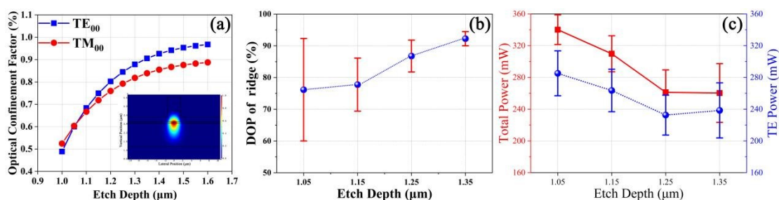
图 2 (a)脊型波导中 TE 00 和 TM 00 模的光限制因子随刻蚀深度的变化;(b)不同刻蚀深度下脊型的偏振度变化趋势;(c)不同刻蚀深度下脊型的总功率和 TE 模式功率变化情况
