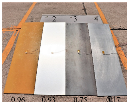
图6 不同种类材料发射率及实物图:1-树脂板,2-阳极氧化铝板,3-钢板,4-镀锌钢板
