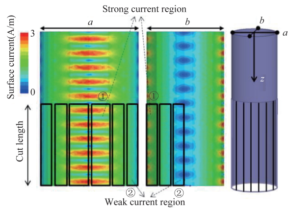
图 2 椭圆波导表面电流分布图, 注: 左侧为长轴方向电流分布, 中间为短轴方向电流分布, 右侧为阶梯型椭圆波导 Vlasov 辐射器示意图, 黑色矩形代表等效隙缝
