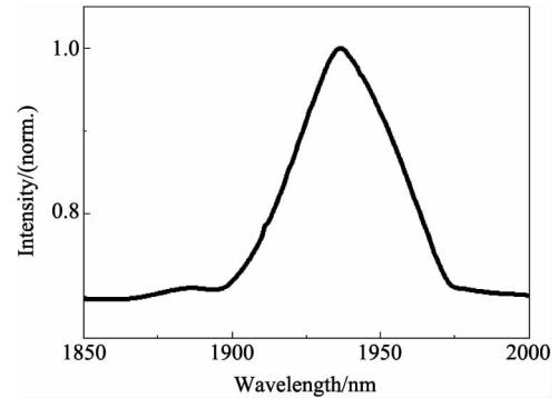
Fig. 3 Optical spectrum of the GaSb-based FP-LD 图 3 砷化镓基法布里-珀罗腔二极管激光器的光谱图
