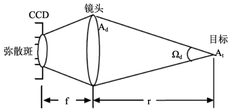
图2 点目标的成像示意图 Fig. 2 Point target imaging diagram
