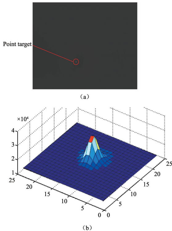
图 6 长波红外试验数据 (a) 长波红外试验图像, (b) 点目标的三维图像
