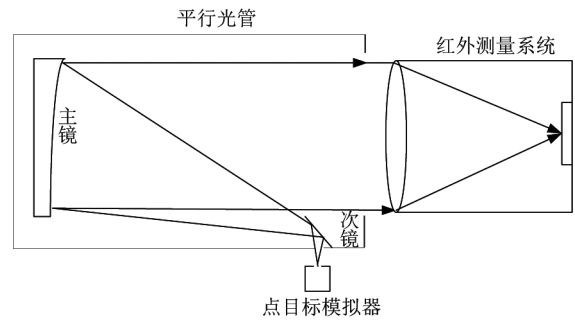
图5 点目标辐射特性测量试验的示意图
