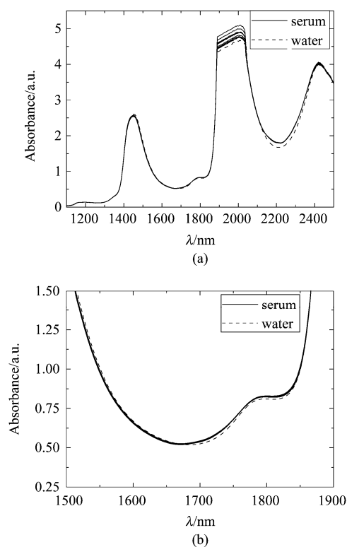
图1 2 mm厚度水与血清的光谱 (a)全谱光谱 (b)一级倍频段光谱
