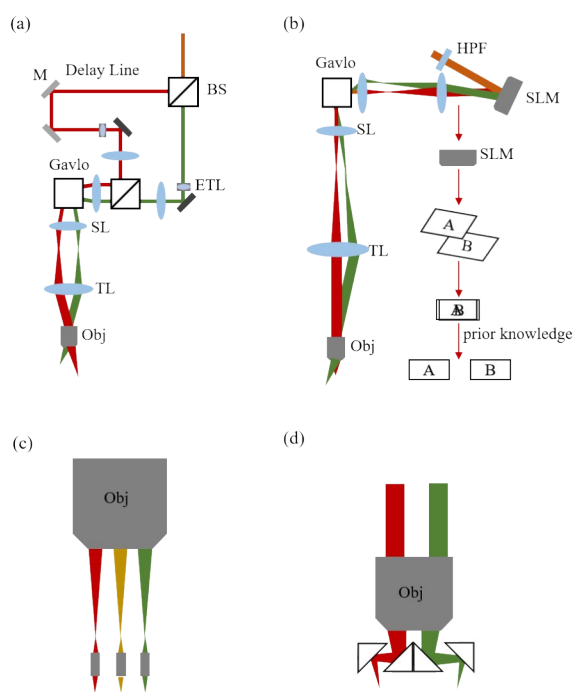
图1 视场分离的实现方式。(a) 发散-偏转法;(b) 相位调制法;(c) 微物镜阵列;(d) 微反射镜模块;BS, 分束镜;M, 反射镜;ETL, 电控可调焦透镜;Gavlo, 振镜;SL, 扫描透镜;TL, 管透镜;Obj, 物镜;HBF, 半波片。
