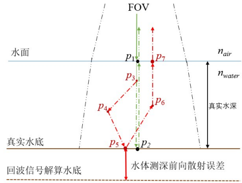
图1 水体前向散射导致的几何误差产生原理
