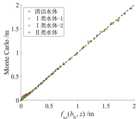
图 5 典型水体前向散射误差蒙特卡罗仿真与修正经验公式 f_{\text{sc}}(b_b, z) 计算结果对比
