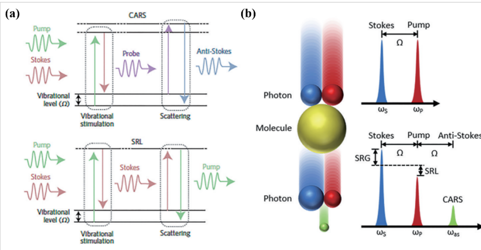
图2 CRS过程的能级变化图及光谱图。(a)CRS过程中的能级变化图,上方为CARS过程,下方为SRS过程。(b)CRS过程中的光谱变化,上方为输入光,下方为输出光。图片引用自文献[2]
