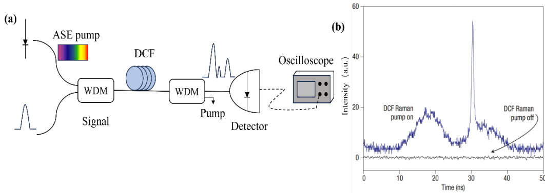
图3 光谱学中放大波长-时间变换的演示。(a)放大波长-时间变换结构示意图。(b)输出结果图。图片引用自文献[18]
