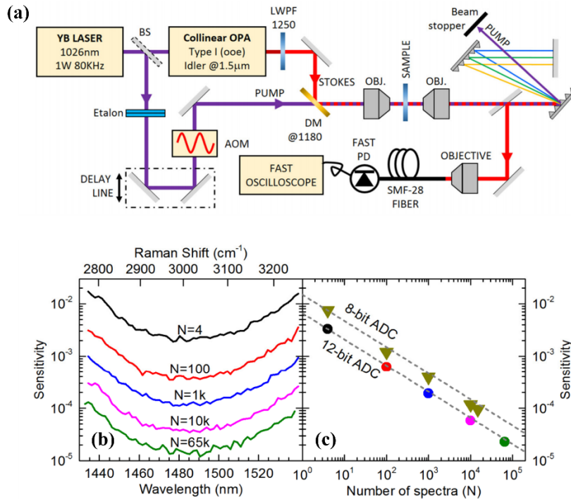
图4 (a)实验装置示意图。(b)用12位示波器测量下的不同光谱数量下SRG的波长相关均方根值和灵敏度。(c)对于8位和12位示波器,SRG的光谱数量与灵敏度函数关系。图片引用自文献[19]
