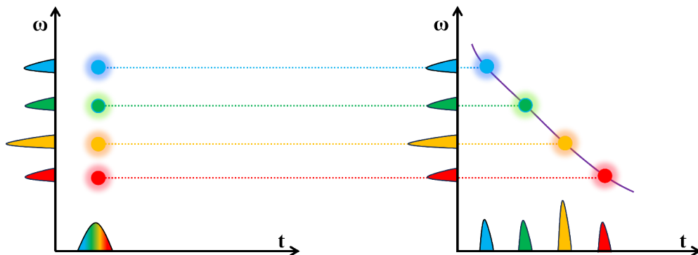
图1 时间拉伸高速测量原理
