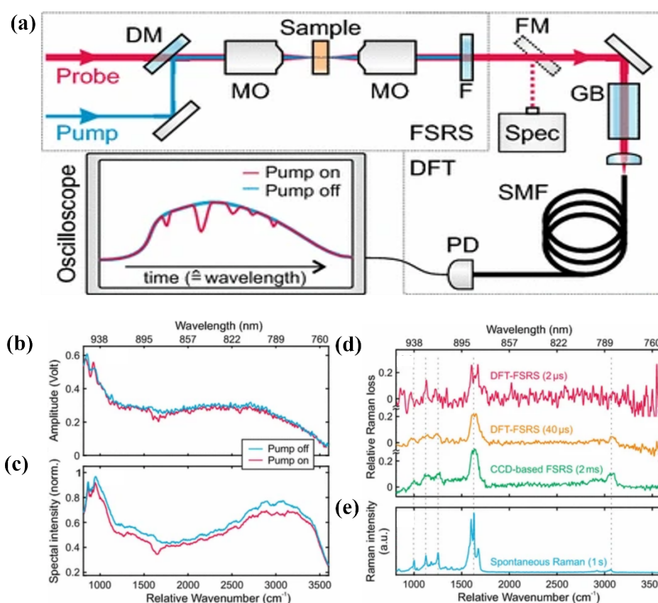
图5 (a)实验装置示意图;(b)使用时间拉伸测量得探测脉冲光谱,分别作为参考泵浦脉冲关闭时(蓝线)和泵浦脉冲开启时的光谱(红线);(c)使用CCD光谱仪测量的探测脉冲光谱,分别作为参考泵浦脉冲关闭时(蓝线)和泵浦脉冲开启时的光谱(红线);(d)时间拉伸获得的单次测量结果(红线)和20次平均测量结果(橙线),以及使用CCD光谱仪获取的结果(绿线);(e)相应的自发拉曼散射光谱。所有测量均在肉桂样品上进行,显著的拉曼峰用垂直线标记,并给出了每种方法的总采集时间。理论采集一张DFT-FSRS光谱时间为1 \mu\text{s} ,采集一张CCD光谱时间为1 ms。图片引用自文献[20]
