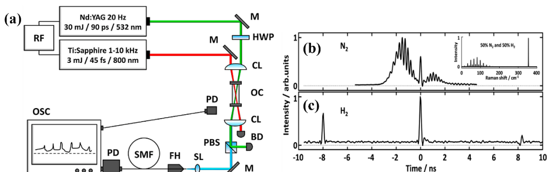
图6 (a)产生振转光谱的实验装置图。以时域波形检测到(b) \text{N}_2 和(c) \text{H}_2 的相干拉曼信号,图中数据为10次瞬时测量的平均值。插图中显示的是在含有50% \text{N}_2 和50% \text{H}_2 的混合物中使用标准化光谱检测方案记录的振转CARS光谱。图片引用自文献[21]
