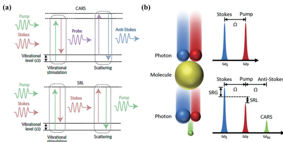
图2 CRS过程的能级变化图及光谱图。(a)CRS过程中的能级变化图,上方为CARS过程,下方为SRS过程。(b)CRS过程中的光谱变化,上方为输入光,下方为输出光。图片引用自文献[2]
