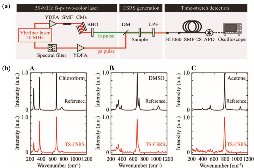
图7 (a)实验装置示意图;(b)分别为(A)氯仿、(B)二甲基亚砷和(C)丙酮的TS-CSRS光谱和自发拉曼散射光谱之间的比较。TS-CSRS光谱的平均值为10000。图片引用自文献[22]
