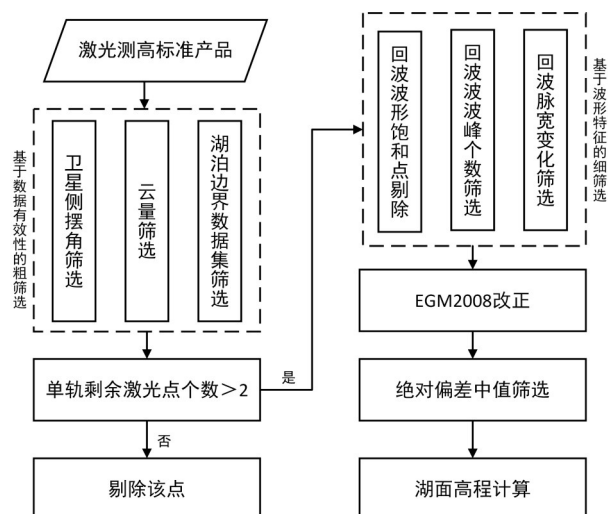
图3 全波体制激光测高数据筛选示意图
