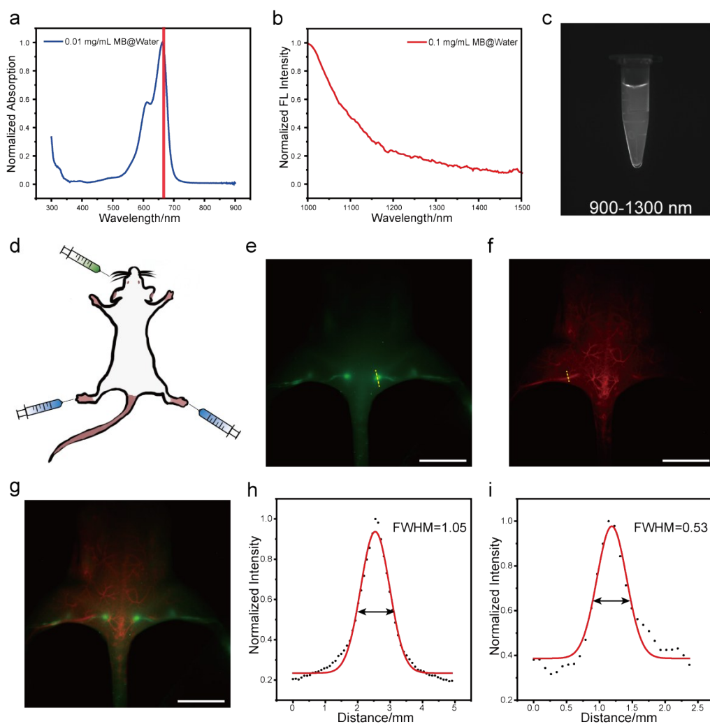
图5 小鼠淋巴结和血管的双通道成像:(a)MB@水溶液(0.01 mg/mL)的归一化吸收光谱。(b)MB@水溶液(0.1 mg/mL)的1000 nm后的归一化发射光谱。(c)在665 nm激光激发下,MB@水溶液(1 mg/mL)在900~1300 nm范围内的荧光成像。(d)小鼠注射操作示意图。(e)小鼠足垫注射MB水溶液,在665 nm激光激发下进行900~1300 nm淋巴结成像的结果。(f)小鼠眼眦注射ICG水溶液,在793 nm激光激发下进行1400~1500 nm血管成像的结果。(g)图(e)与图(f)的融合双通道图像。(h)沿着图(e)中黄色虚线处淋巴结的截面荧光强度分布。(i)沿着图(f)中黄色虚线处血管的截面荧光强度分布。比例尺:10 mm。
