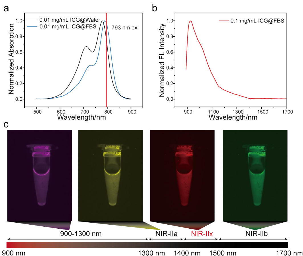
图2 ICG 的光学特性表征:(a)ICG@FBS 溶液 (0.01 mg/mL) 和 ICG@水溶液 (0.01 mg/mL) 的归一化吸收光谱。(b)ICG@FBS 溶液 (0.1 mg/mL) 的归一化发射光谱。(c)在 793 nm 激光激发下,ICG@FBS 溶液 (0.1 mg/mL) 在 900~1300 nm、1300~1400 nm、1400~1500 nm 和 1500~1700 nm 范围内的荧光成像。
