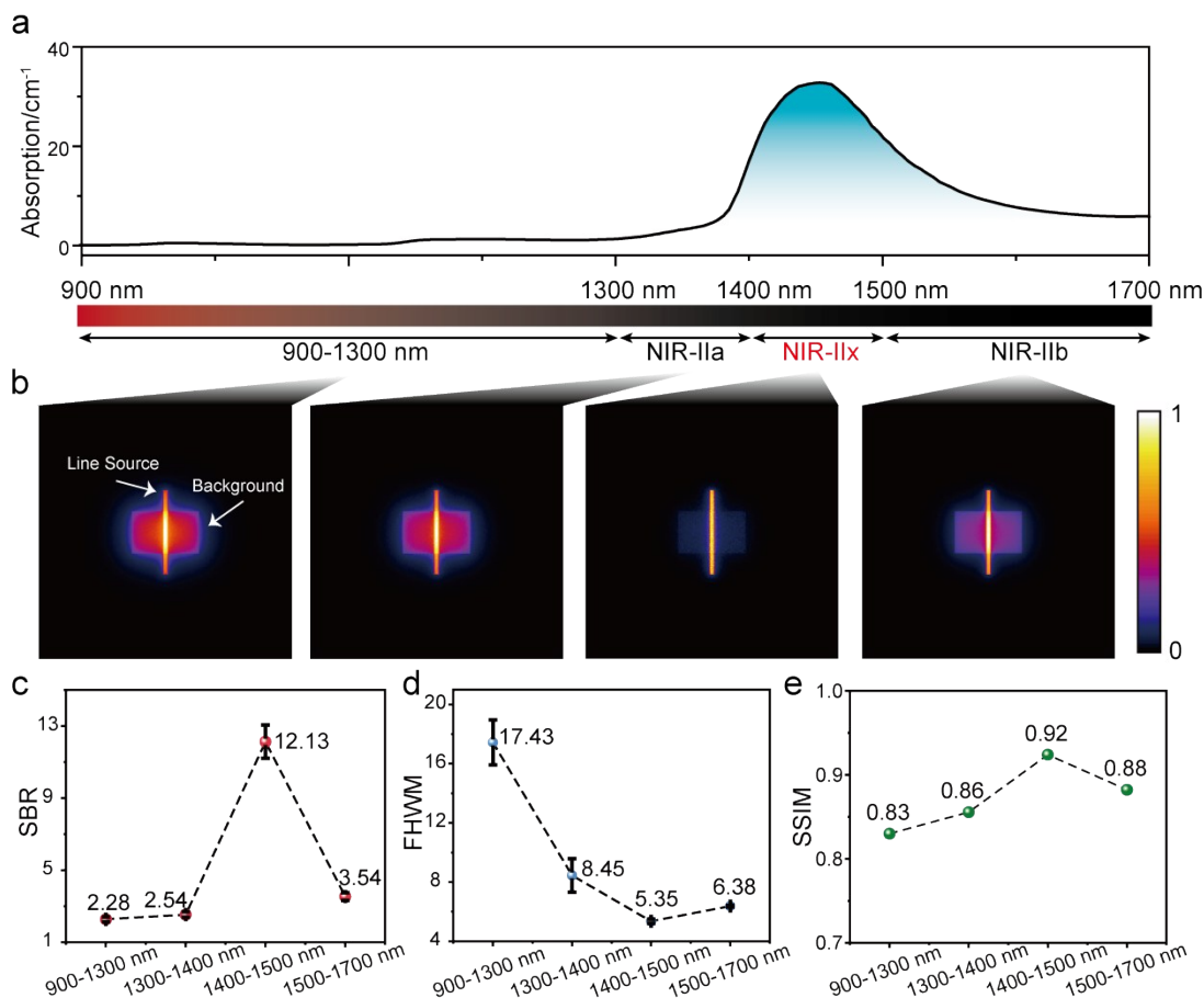
图 1 NIR-II 生物成像的 Monte Carlo 仿真结果:(a)水在 900~1700 nm 的吸收光谱。(b)模拟 900~1300 nm、1300~1400 nm、1400~1500 nm、1500~1700 nm 的成像仿真结果(样品深度为 1 mm)。(c)对(b)中模拟图像进行 SBR 分析的结果。(d)对(b)中模拟图像进行 FWHM 分析的结果。(e)对(b)中模拟图像进行 SSIM 分析的结果。
