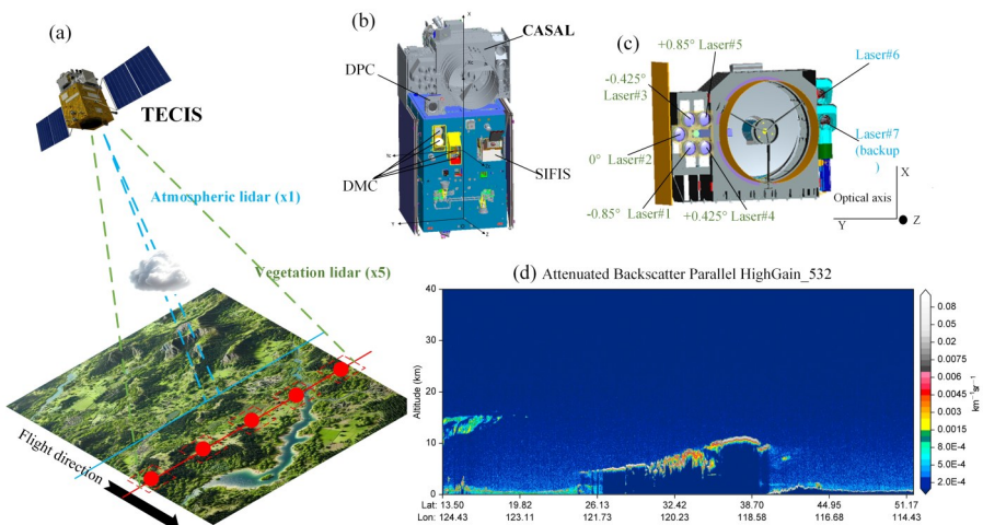
图1 陆地碳监测卫星介绍:(a) 卫星观测示意图;(b) 卫星载荷分布;(c) 多波束激光雷达相机光轴结构;(d) 532 nm平行通道高增益模式数据
