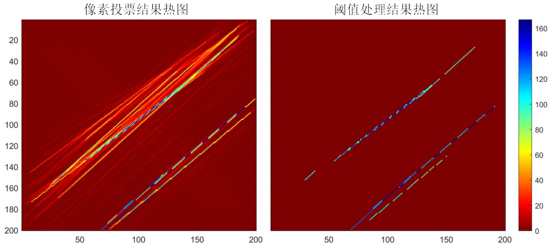
图3 像素投票与阈值处理
