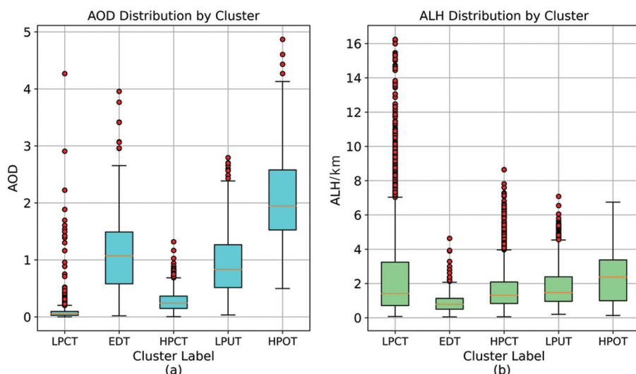
图5 由GMM获取的5个聚类结果:(a)AOD分布;(b)ALH分布
