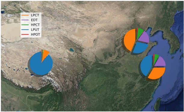
图8 气溶胶剖面聚类在中国地区的地域分布特征 Fig. 8 Geographical distribution characteristics of aerosol profile clustering in China
