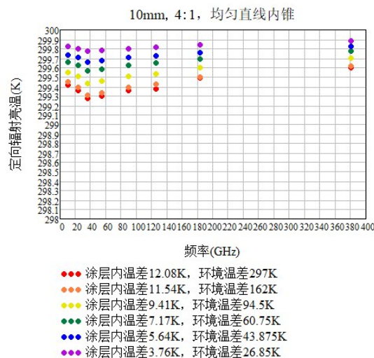
图5 不同环境温度条件下,均匀涂覆锥体定标源的定向辐射亮温 10 mm 周期锥体(基底温度 T_{\text{基底}}=300\text{ K} ,环境背景亮温低于定标源基底温度,因此定标源辐射亮温值偏低。)
