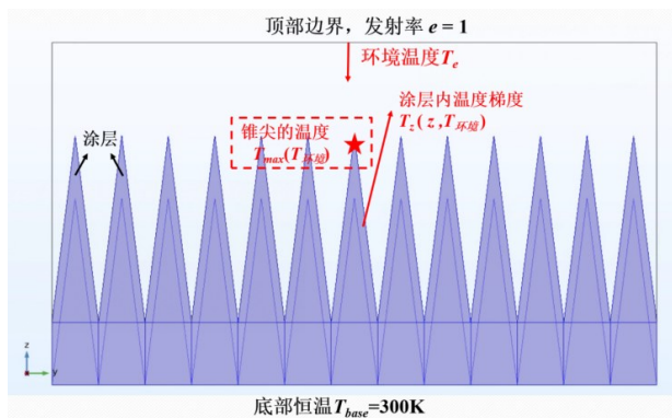
图3 针对定标源涂层内温度分布的热仿真场景设置示意图
