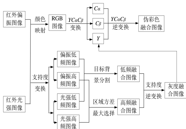
图 17 文献[54]的算法原理图
