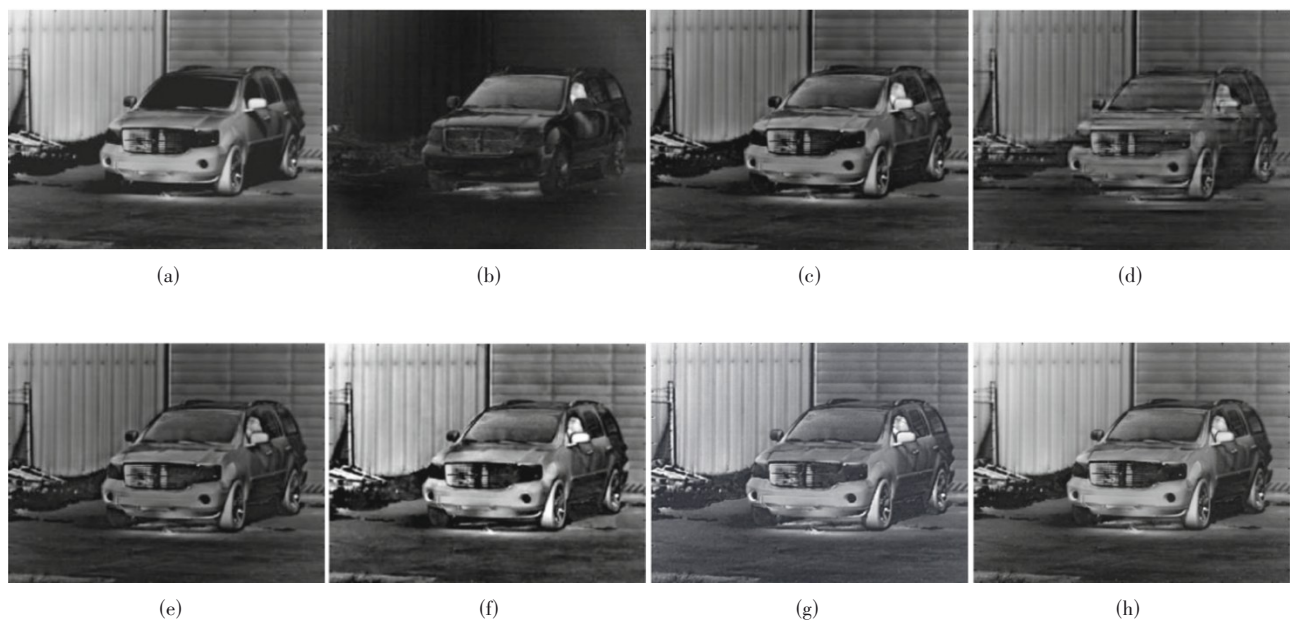
图 10 不同数学/统计学融合算法对比:(a)强度图像,(a)强度图像;(b)偏振度图像;(c)LP;(d)DWT;(e)NSCT;(f)文献[27];(g)文献[28];(h)文献[29]
