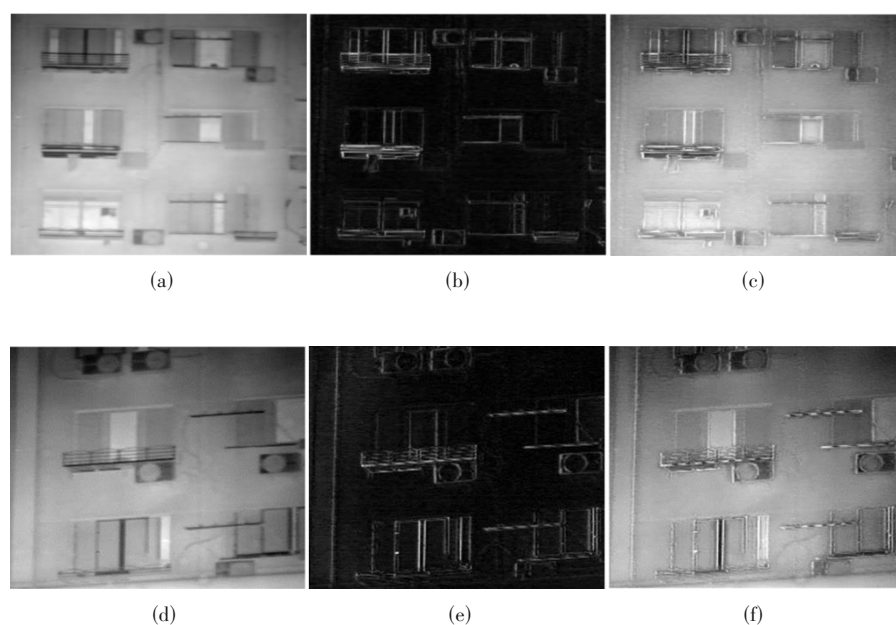
图7 不同塔形分解融合算法对比:(a)强度图像;(b)偏振度图像;(c)文献[10], (d)强度图像;(e)偏振度图像, (f)文献[12]
