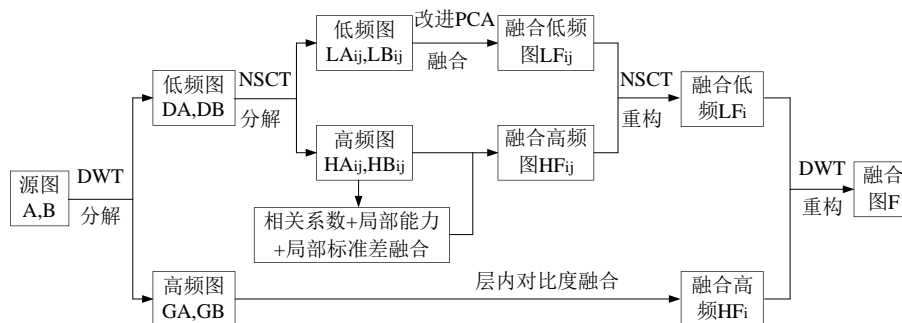
图 20 DWT、NSCT和改进PCA协同的图像融合过程 [56]
