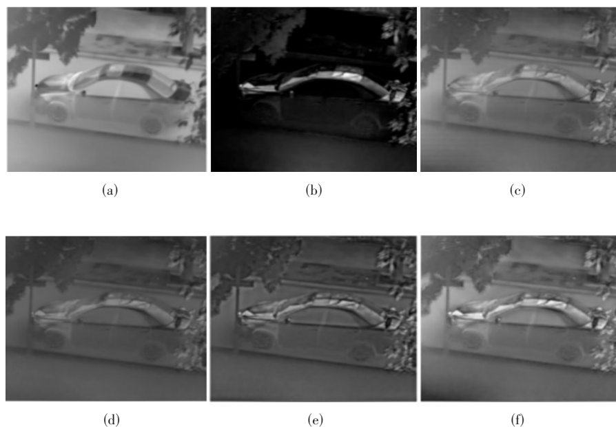
图 21 嵌接式融合算法对比:(a)强度图像:(b)偏振图像(a)强度图像:(b)偏振图像:(c)改进PCA;(d)DWT-PCA;(e)NSCT-DWT;(f)文献[56]
