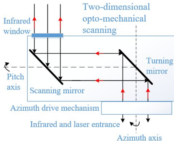
Fig. 3 Principle diagram of light beam control subsystem 图3 光束控制分系统原理示意图
