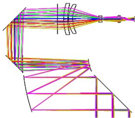
Fig. 13 Fine track module optical path diagram 图13 精跟踪模块光路图
