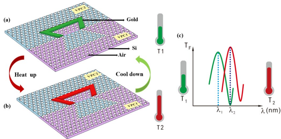
图1 能谷光子晶体MZI热光调制器结构示意图及干涉峰位移示意图:低温(a)和高温(b)分别为绿色和红色表,紫色和蓝色分别表示VPC1和VPC2;(c)温度变化引起的干涉峰位移示意图,其中 \lambda_1 和 \lambda_2 分别对应 T_1 和 T_2 温度下干涉峰的位置, T_F 为电光调制器的正向透射率。
