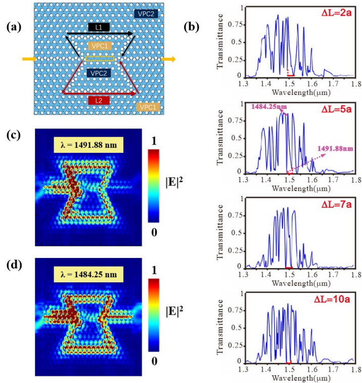
图3 能谷光子晶体 MZI 结构及光路示意图、透射率光谱曲线及电场强度分布:(a)能谷光子晶体 MZI 结构及光路示意图( \Delta L = 5a ); (b) \Delta L = 2a, 5a, 7a, 10a 时的透射率光谱曲线; (c) (d) 分别为当 \Delta L = 5a 时, MZI 在 1491.88 \text{ nm} 和 1484.25 \text{ nm} 处的电场强度分布(相应位置已在图 b 标出)。
