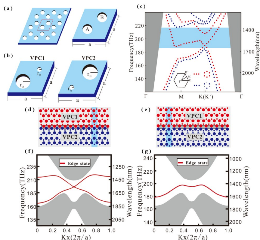
图2 结构参数示意图和光子能带图:(a)初始光子晶体结构参数示意图。平行四边形表示由两个空气孔(A和B)组成的蜂窝晶格,其中晶格常数 a = 0.44\text{ }\mu\text{m} ,圆半径 r = 0.08\text{ }\mu\text{m} ,硅基板厚度 h = 0.22\text{ }\mu\text{m} ;(b)VPC1(左)和VPC2(右)的结构示意图;(c)初始蜂窝PC(红色虚线)和VPC1(蓝色虚线)的光子能带图,蓝色矩形区域为带隙,灰色阴影为空气锥;(d)和(e)由VPC1和VPC2组成的锯齿形和胡须形边界的几何形状;(f)和(g)由VPC1和VPC2组成的锯齿形和胡须形边界的边缘状态能带图,所用的超元胞为(d)和(e)中的蓝色矩形区域。
