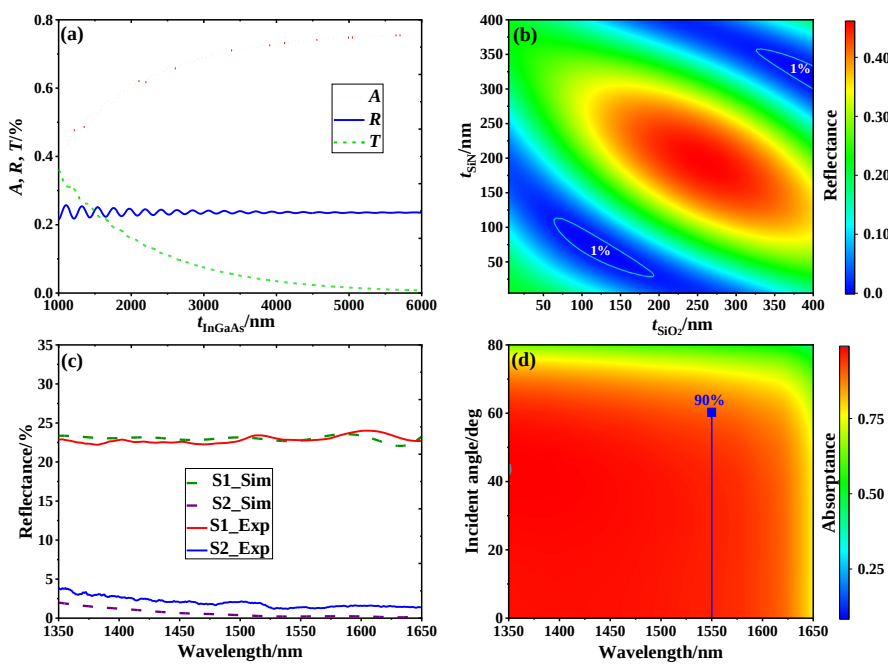
图4 光学仿真结果和实验结果:(a) \lambda=1\,550\,\text{nm} 时,无减反层器件吸收率( A )、反射率( R )、透射率( T )随吸收层厚度 t_{\text{InGaAs}} 的变化关系图;(b) t_{\text{InGaAs}}=4\,050\,\text{nm} , \lambda=1\,550\,\text{nm} 时,器件的反射率随减反射层 \text{SiO}_2 和 \text{SiN} 厚度的变化关系图;(c)器件反射谱的计算与实验结果对比图,S1为沉积了 \text{SiO}_2/\text{SiN} 减反射层的样品,S2为未沉积减反射层的样品;(d) t_{\text{InGaAs}}=4\,050\,\text{nm} , t_{\text{SiO}_2}=140\,\text{nm} , t_{\text{SiN}}=60\,\text{nm} 时,器件吸收率随激光波长和入射角度变化图
