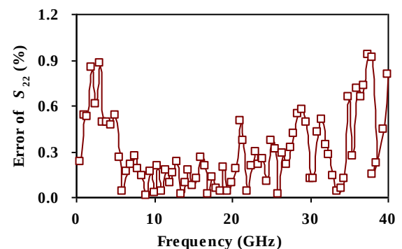
(d) S_{22}
