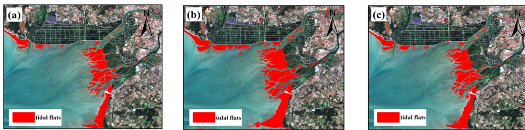
图 7 三种分类方法潮滩结果图:(a)最小距离法;(b)极大似然法;(c)支持向量机
