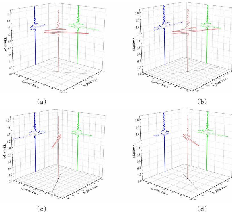
图2 阵列天线的线偏振太赫兹波调控
