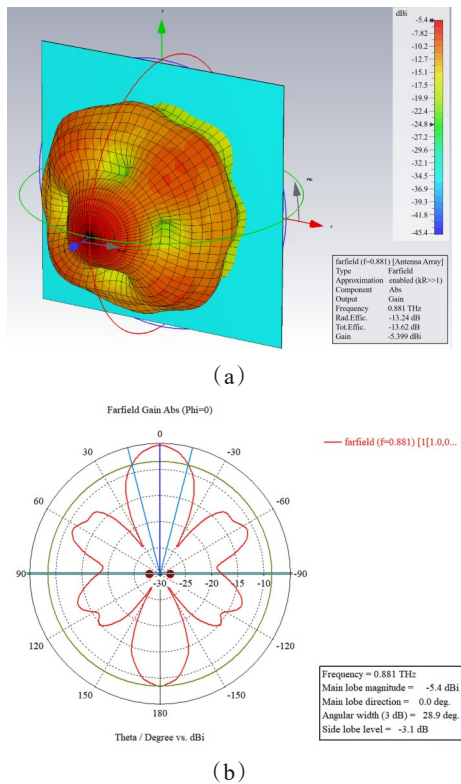
图6 天线阵列的增益和方向图仿真结果
