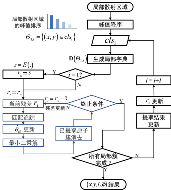
图4 SOMP算法流程
