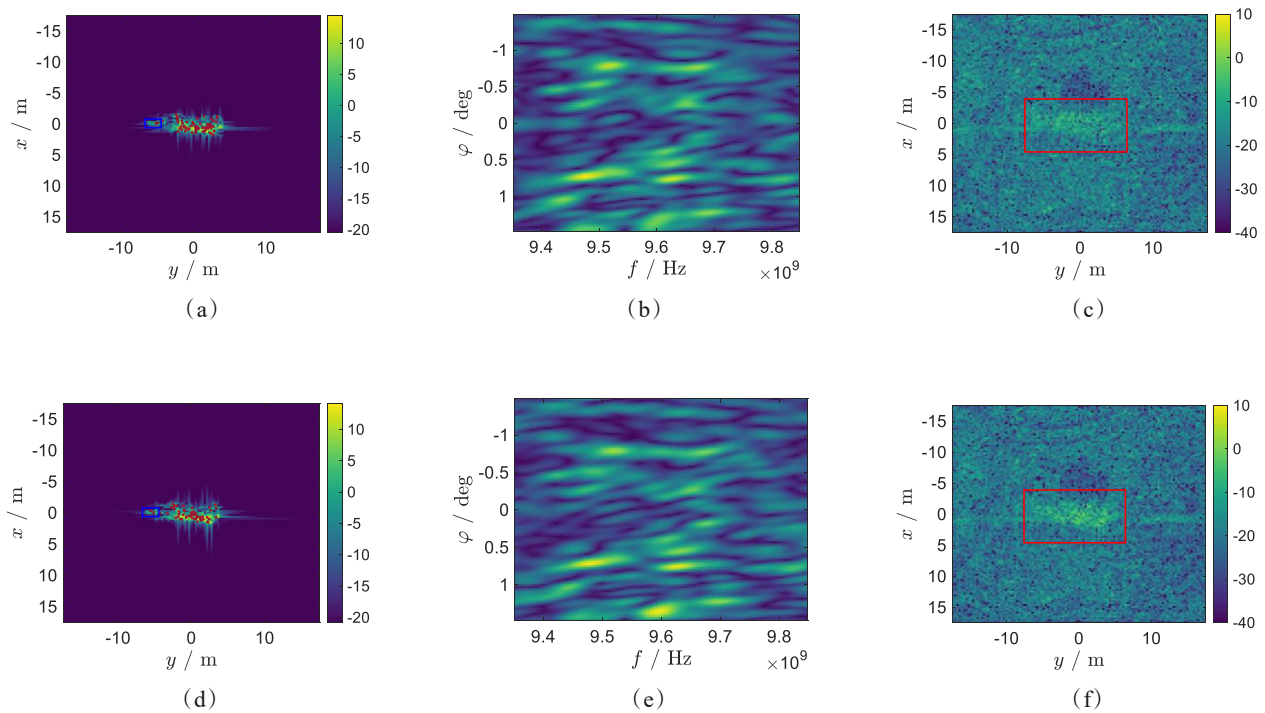
图12 SOMP算法和OMP算法对MSTAR中T62的属性散射中心提取结果:(a)OMP重建SAR图像;(b)OMP重建频率域图像;(c)OMP重建结果的残差图像;(d)SOMP重建SAR图像;(e)SOMP重建频率域图像;(f)SOMP重建结果的残差图像
