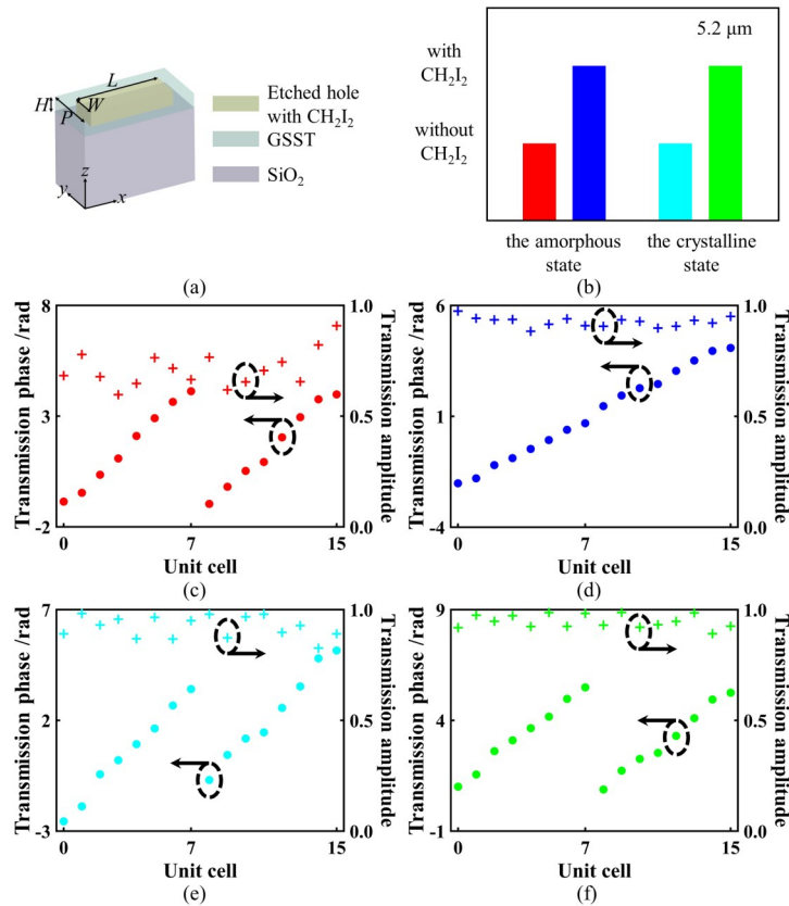
图2 超单元结构及其在不同相变状态下的可调特性:(a)超单元示意图,参数分别为 H=2\ \mu\text{m} , P=1\ \mu\text{m} , W 从0变化到 1\ \mu\text{m} , L 从0变化到 10\ \mu\text{m} ;(b)可调编码超表面的四个状态;非晶态GSST的编码超单元在刻蚀孔中(c)没有或者(d)有 \text{CH}_2\text{I}_2 液体的透射系数和相移;晶态GSST的编码超单元在刻蚀孔中没有(e)或者有(f) \text{CH}_2\text{I}_2 液体的透射系数和相移,以上说明了编码超单元在不同相变状态时的可调特性
