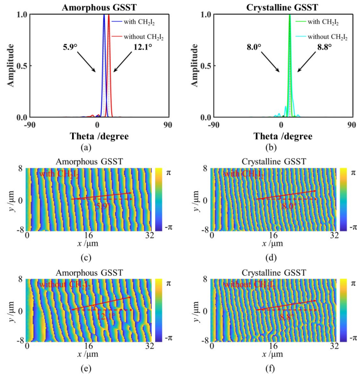
图3 可调编码超表面的偏折功能:(a)当GSST处于非晶态、波长为 5.2\ \mu\text{m} 时,刻蚀孔中有(蓝色线)或者没有(红色线) \text{CH}_2\text{I}_2 液体的模拟远场散射图;作为对照,晶态GSST的散射图展示在(b)中;非晶态GSST刻蚀孔中有(c)或者没有(e) \text{CH}_2\text{I}_2 液体在 xy 平面的相位分布;晶态GSST刻蚀孔中有(d)或者没有(f) \text{CH}_2\text{I}_2 液体在 xy 平面的相位分布。这些结果说明了可调编码超表面在不同条件下的偏转特性
