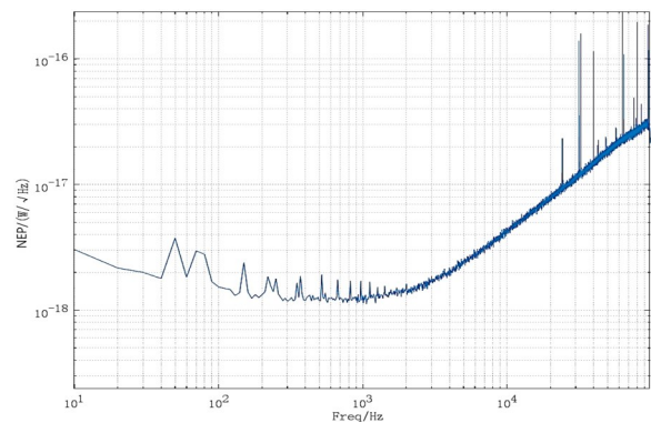
Fig 22 NEP result of KIDs 图 22 KIDs 的 NEP 结果图
