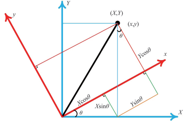
Fig. 8 Diagram of coordinate rotation formula 图 8 坐标旋转公式图示
