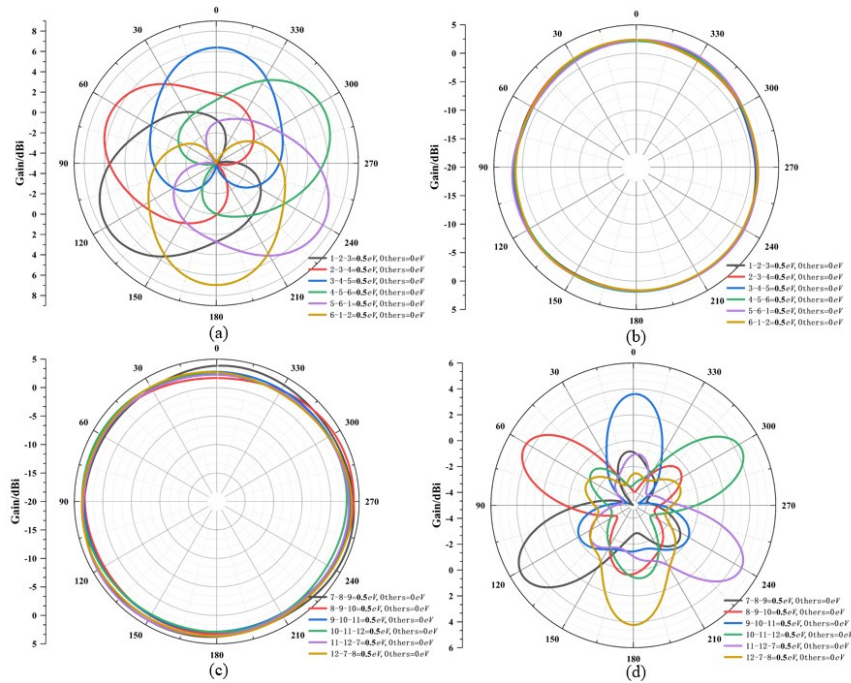
Fig. 7 Radiation direction of 1.08 THz and 1.58 THz; (a)-(b) Mode 1-6; (c)-(d) Mode 7-12 图7 1.08 THz和1.58 THz上的辐射方向图;(a)-(b)模式1-6;(c)-(d)模式7-12
