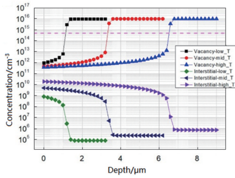
图2 不同温度结深推进结果
