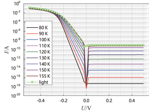
图3 高温结构不同温度暗电流与光电流模拟结果
