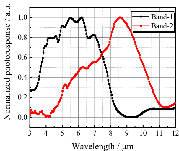
图8 长/长波双色超晶格探测器光谱响应曲线
