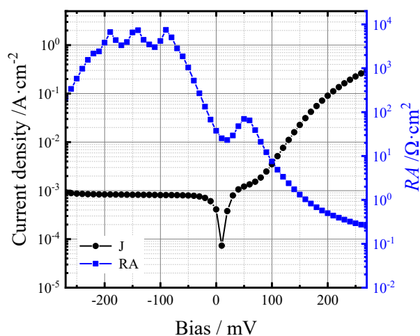
图7 J - V 和 RA - V 特性曲线
