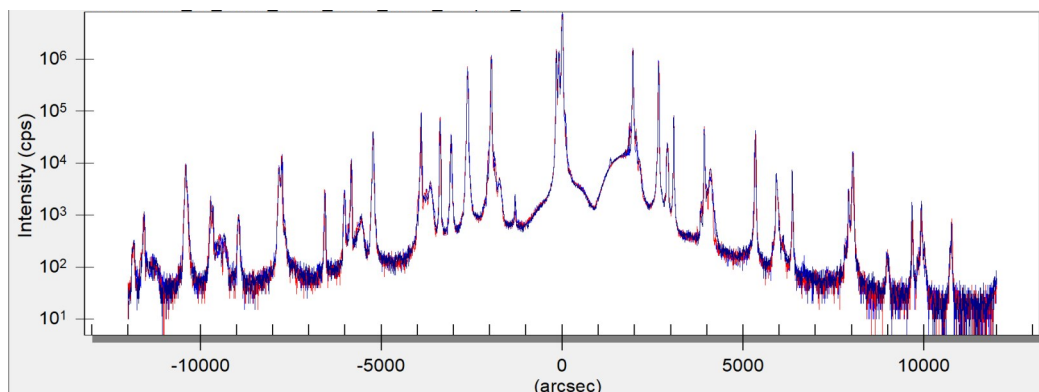
图5 长/长波双色超晶格材料 XRD 测试图谱
