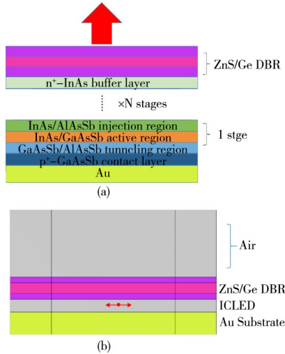
图1 (a)谐振腔带间级联LED结构示意图,(b)谐振腔LED仿真结构示意图
