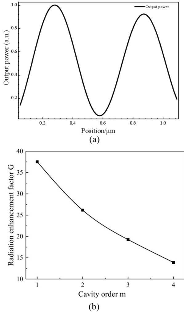
图4 (a)腔长为 \lambda 时,谐振腔LED输出功率与偶极子在腔内位置的关系,(b)辐射增强因子 G 与腔阶 m 的关系
