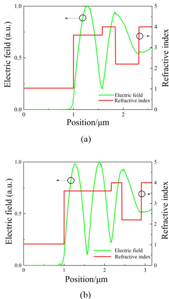
图3 不同腔长下的谐振腔内部电场强度分布:(a) \lambda/2 , (b) \lambda
