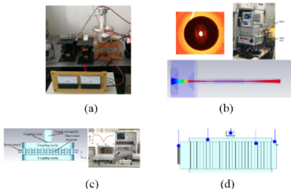
图 17 梯形慢波结构扩展相互作用振荡器
