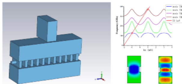
图 20 谐波扩展相互作用振荡器结构及色散情况
