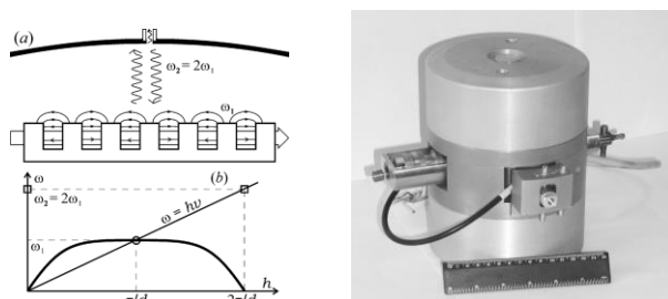
图 37 超辐射奥罗管原理示意图及装配示意图
