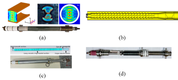
图 29 创新结构回旋振荡器及放大器 Fig. 29 Innovative structure Gyrotron and Gyrotron amplifier
