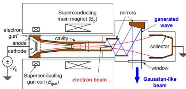
图 25 回旋管结构示意图 Fig. 25 The schematic diagram of Gyrotron structure
