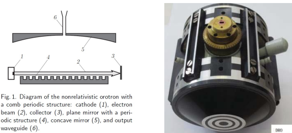
图 35 W 波段奥罗管及实物示意图
