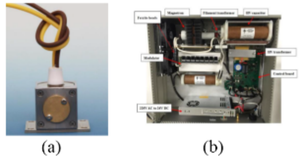
图 30 两种 W 波段空间谐波磁控管 Fig. 30 Two types of W-band spatial harmonic Magnetrons
