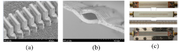
图6 新型太赫兹螺旋慢波线结构 Fig. 6 Novel terahertz spiral interaction structure
