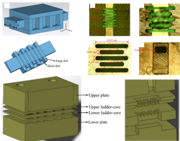
图 24 长短槽梯形慢波结构 Fig. 24 Unequal-length Slots interaction structure
