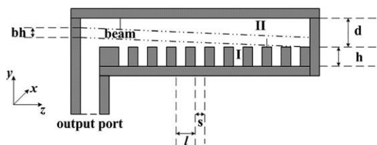
图 32 斜注管原理示意图
