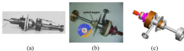
图 26 脉冲磁场回旋管 Fig. 26 Pulsed magnetic field Gyrotron
