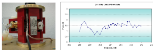
图 19 0.264 THz 扩展相互作用振荡器
