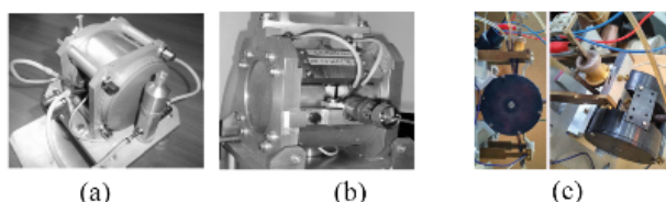
图 34 0.346 THz斜注管实验研究
