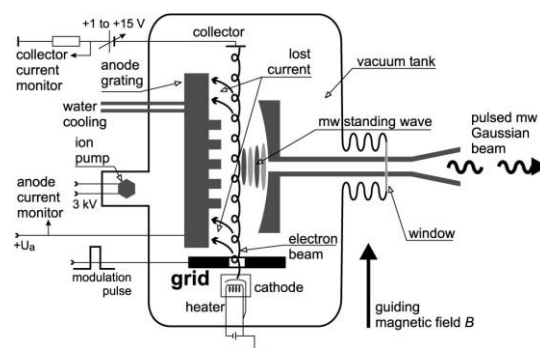
图 36 超辐射奥罗管结构示意图
