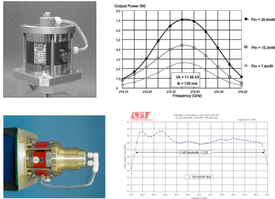
图 21 G 波段及 W 波段扩展相互作用速调管 Fig. 21 G-band and W-band Extended Interaction Klystron
