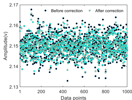
图 18 谐波信号的峰值波动
