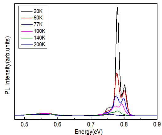
图 1 掺杂面密度为 1.14\times 10^{12}\text{ cm}^{-2} 的 SQW 变温 PL 光谱
