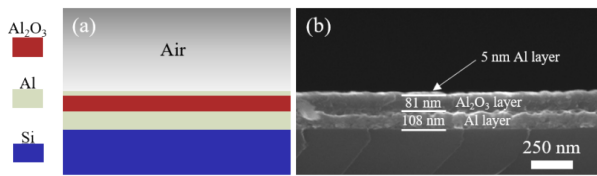
图2 三层薄膜堆栈结构的吸收器 (a) 结构示意图, (b) SEM截面图
