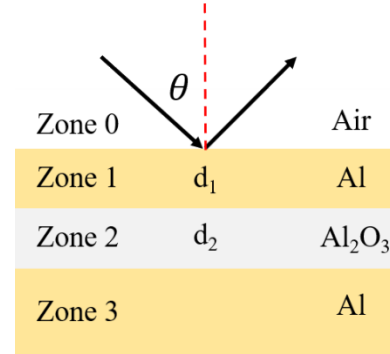
图4 吸收器结构示意图
