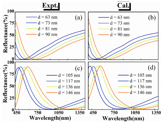
图3 吸收器的反射光谱曲线 (a) Al 2 O 3 厚度分别为63 nm、73 nm、81 nm、90 nm样品的实验反射光谱曲线, (b) Al 2 O 3 厚度分别为63 nm、73 nm、81 nm、90 nm样品的模拟反射光谱曲线, (c) Al 2 O 3 厚度分别为105 nm、117 nm、136 nm、146 nm样品的实验反射光谱曲线, (d) Al 2 O 3 厚度分别为105 nm、117 nm、136 nm、146 nm样品的模拟反射光谱曲线
