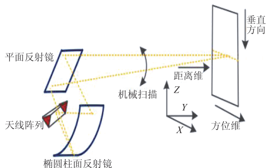
图1 340GHz 安检成像系统结构
