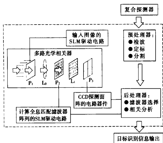
图 1 光电混合自动目标识别系统的基本工作原理框图
